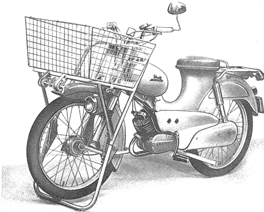
Abb. 1 Rabeneick-Lastenmoped Typ Lastboy
